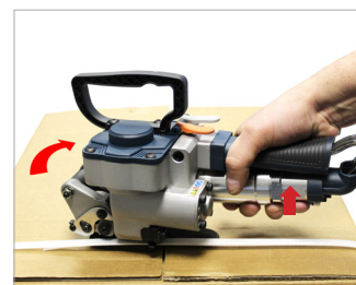
Sgancio della reggetta tramite leva Strap outfeed by lever
